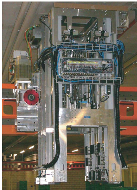
Detailansicht Gebindegreifsystem.
