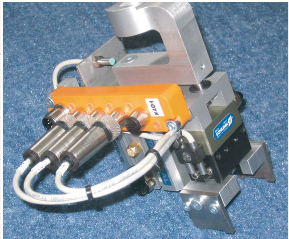
Pickergreifer zum verpacken von Kleinteilen in weniger als 1 Sekunde.
