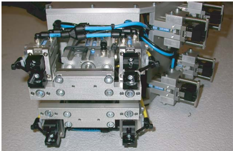
Einlege-/Ent- nahmegreifer vierfach für Alu-Teile.
