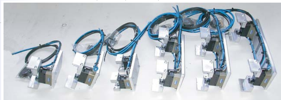
Entnahmegreifer für Kunststoffteile einfach oder zweifach.
