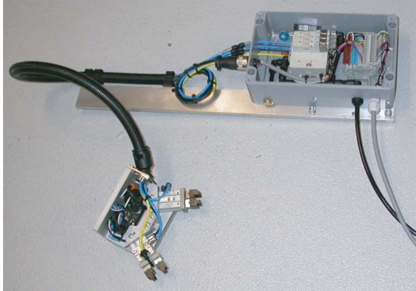
Einlege-/Ent- nahmegreifer zweifach für Alu-Teile mit Wechselsystem.
