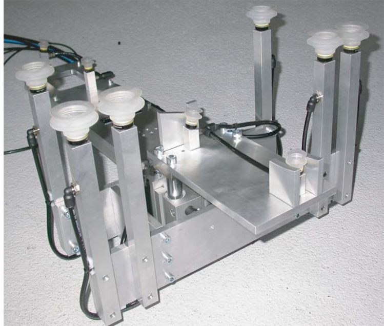
Umsetz-/Ent- nahmgreifer für 2-Komponenten Kunststoffteile mit Andock- und Aufschiebehub.
