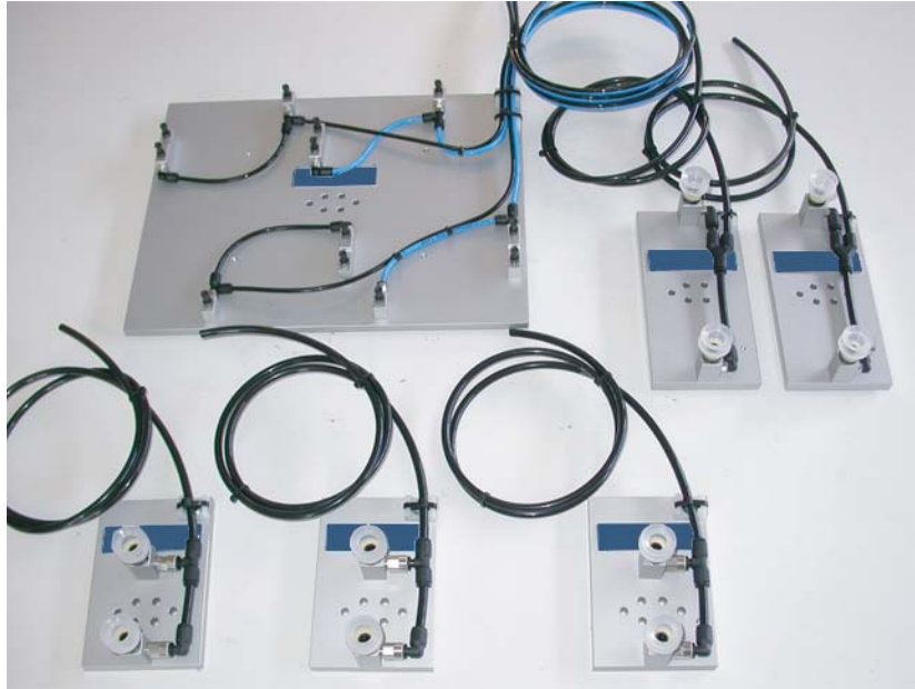
Vakuumgreifer für Kunststoffteile einfach oder mehrfach.
