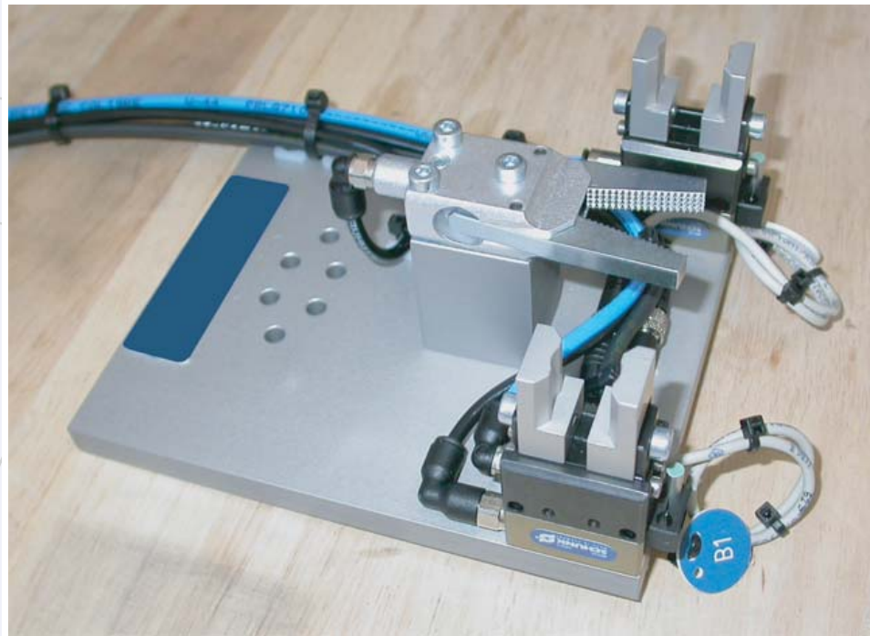
Entnahmegreifer für zwei Kunststoffteile mit Anguss.
