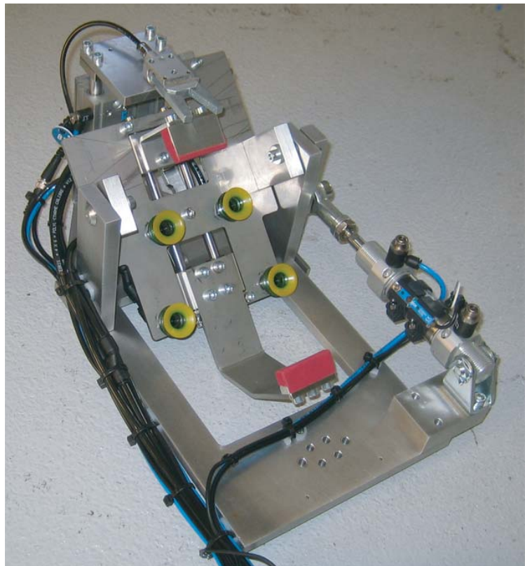
Entnahmegreifer zum Entformen und Entnehmen von Kunststoffteil mit Anguss.
