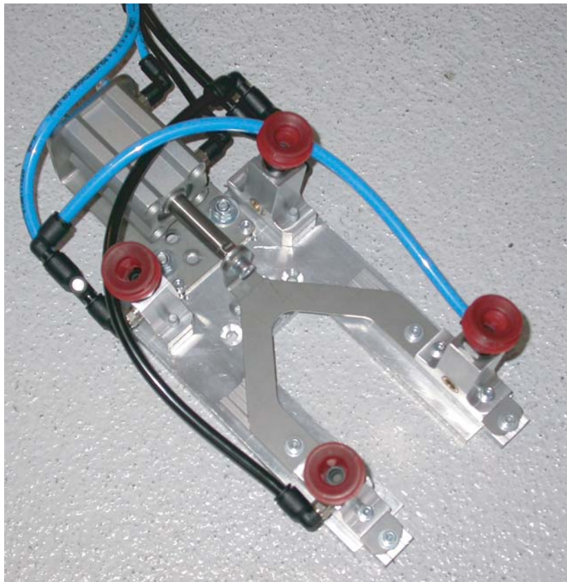
Vakuumgreifer für vier Kunststoffteile mit Spreizhub.
